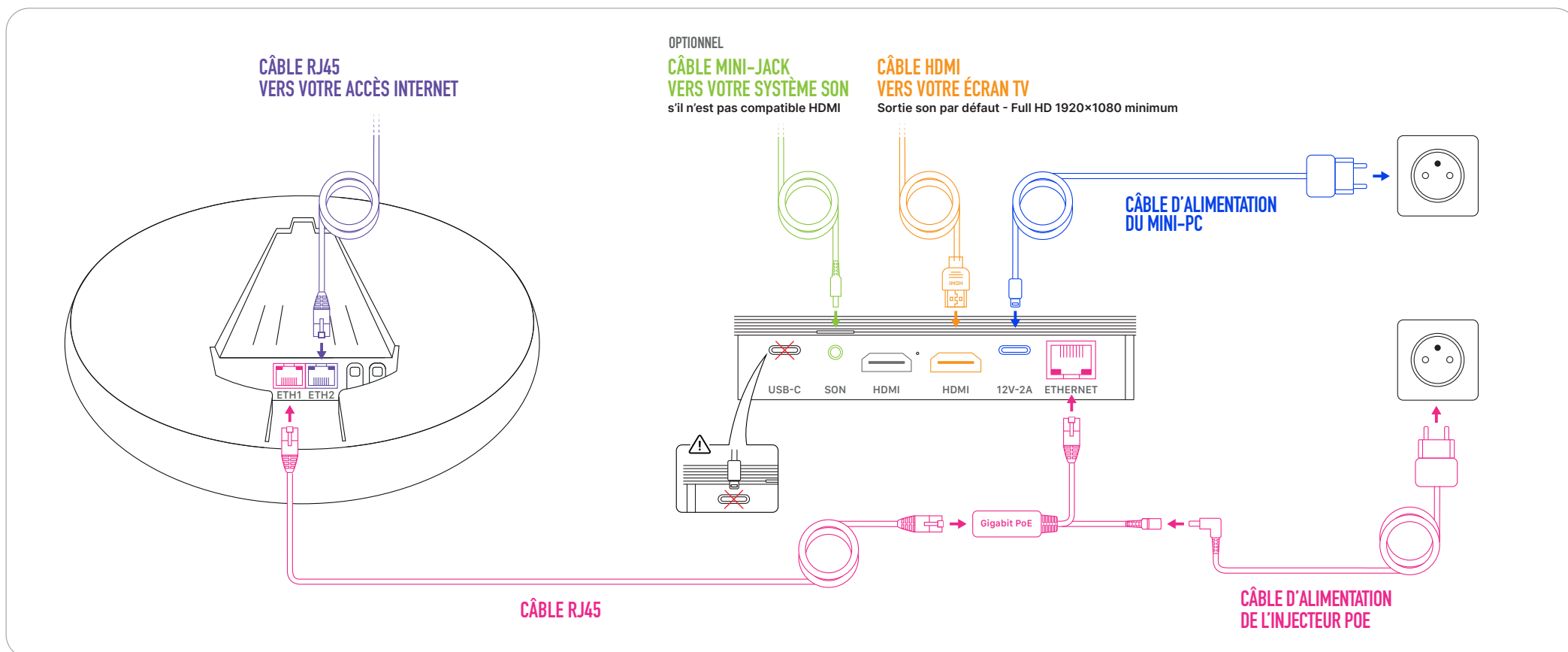
Câble d'alimentation injecteur PoE
